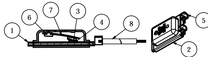
A-A section
